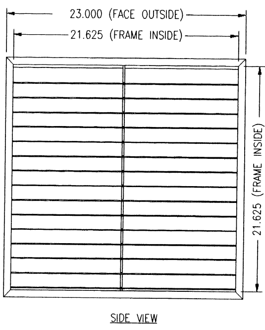
② LOUVER ASSEMBLY SCALE: NONE
