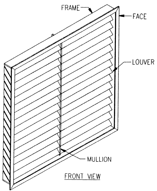
① LOUVER ASSEMBLY SCALE: NONE
