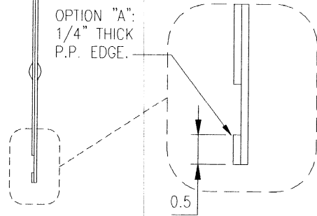
A SECTION SCALE: N.T.S.
