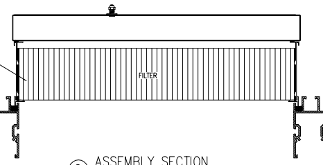
C ASSEMBLY SECTION SCALE: 1:3
