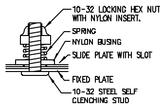
4 CLAMP STUD DETAIL
