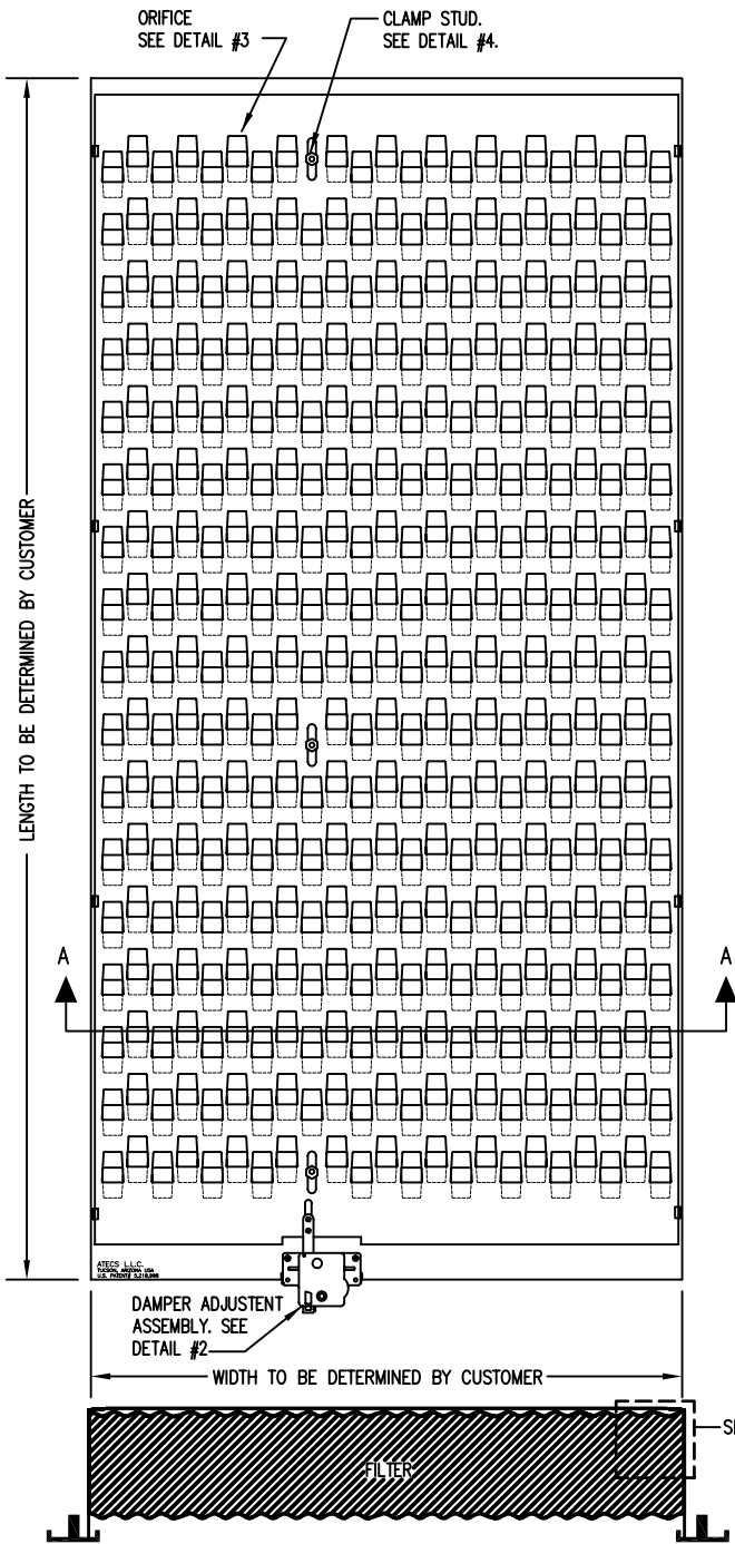
SECTION A-A
